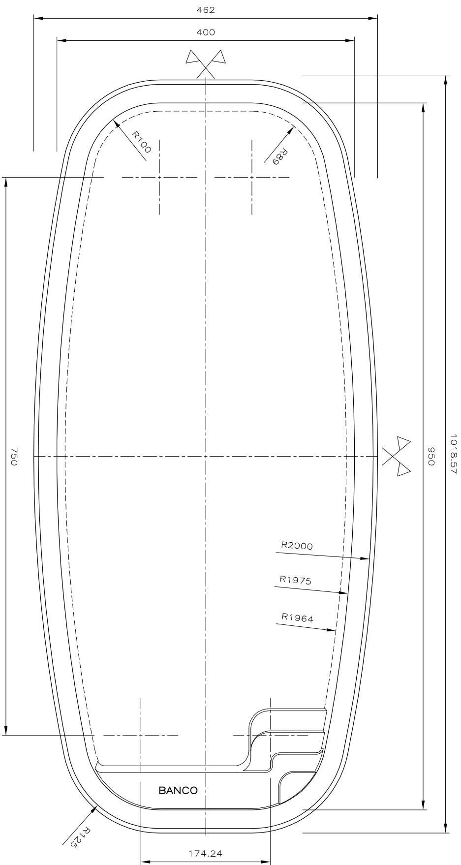
Vista Superior Escala 1/50
